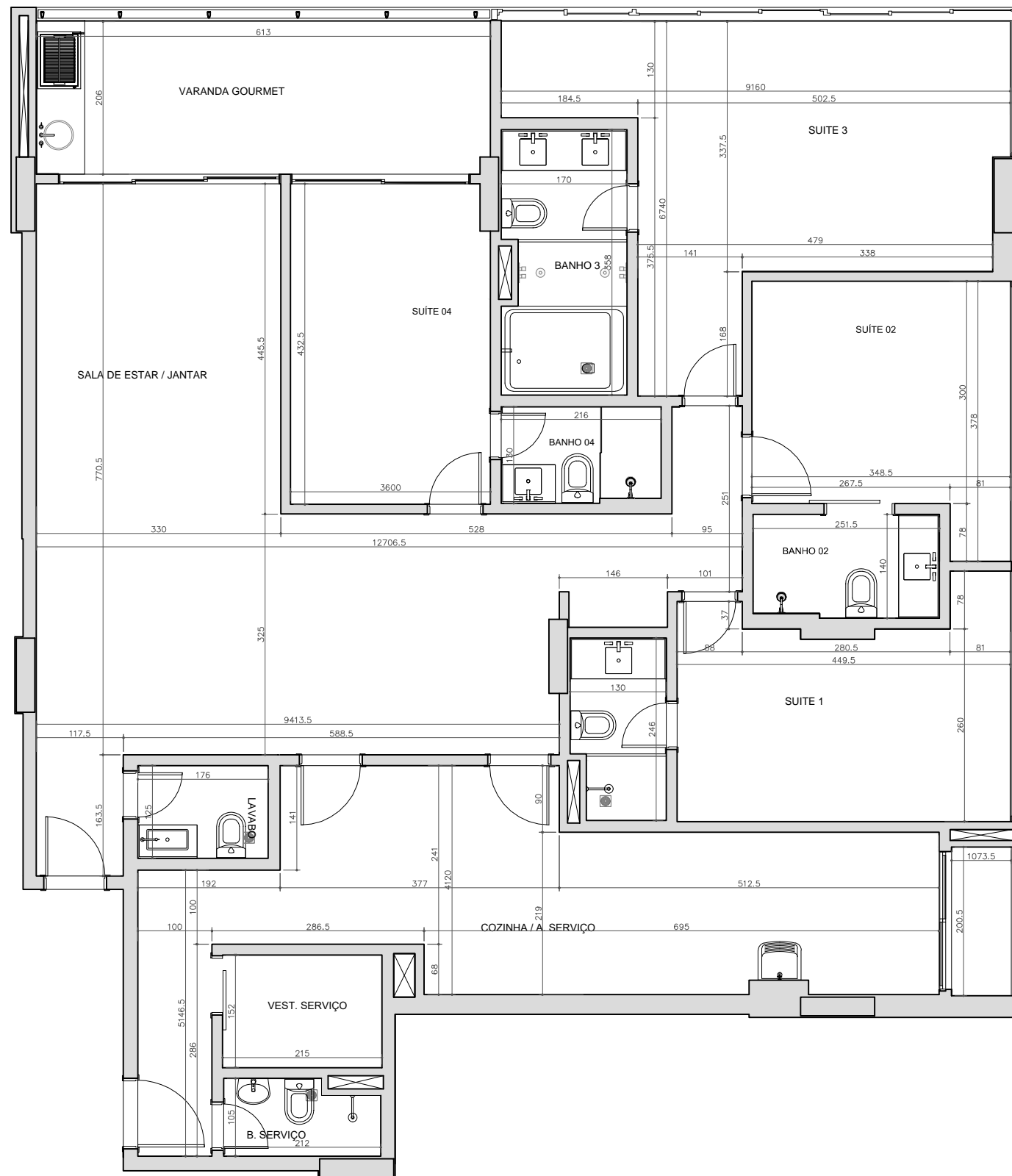
FINAIS 02 E 06 ESC. 1:75
