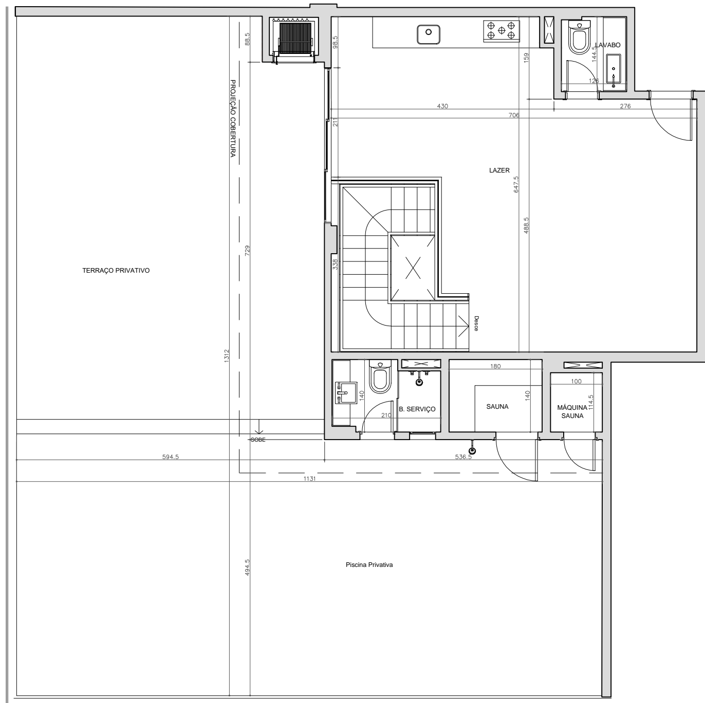
UNIDADE 606 - PAV. SUPERIOR ESC. 1:75
