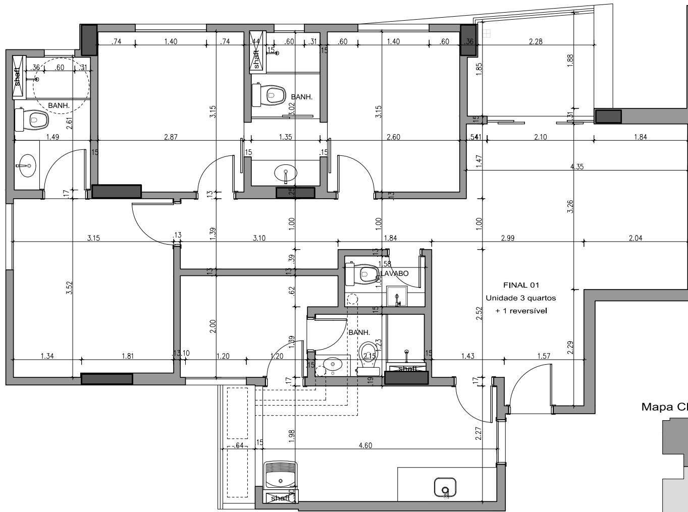
Planta referente aos pavimentos ímpares: 1º, 3º, 5º, 7º, 9º e 11º.
